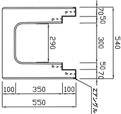
断面図
