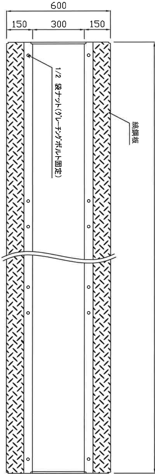
上面図
