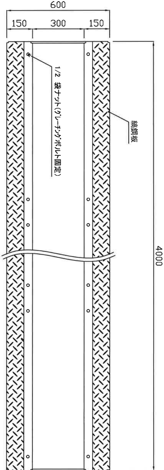
上面図
