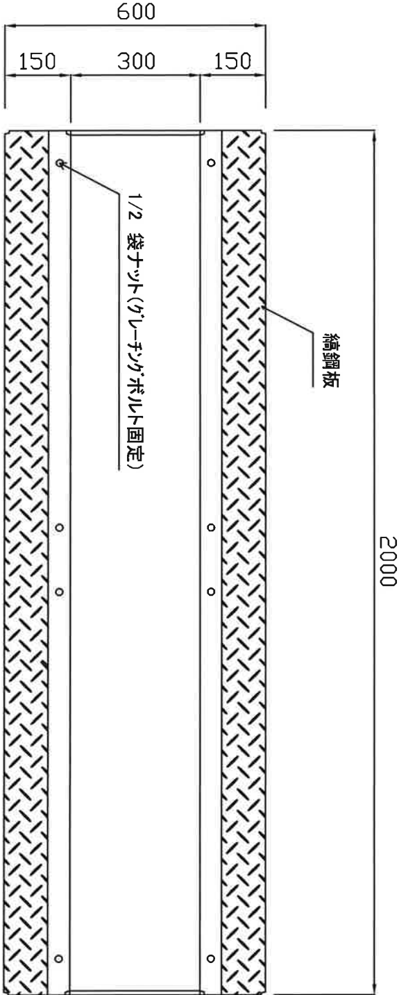
上面図
