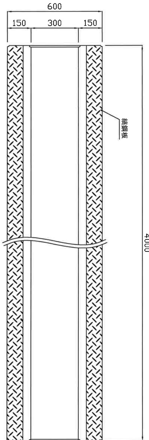
上面図
