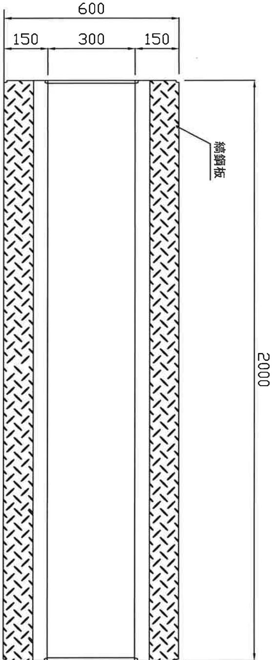
上面図
