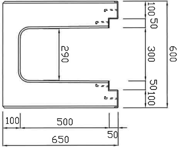
断面図
