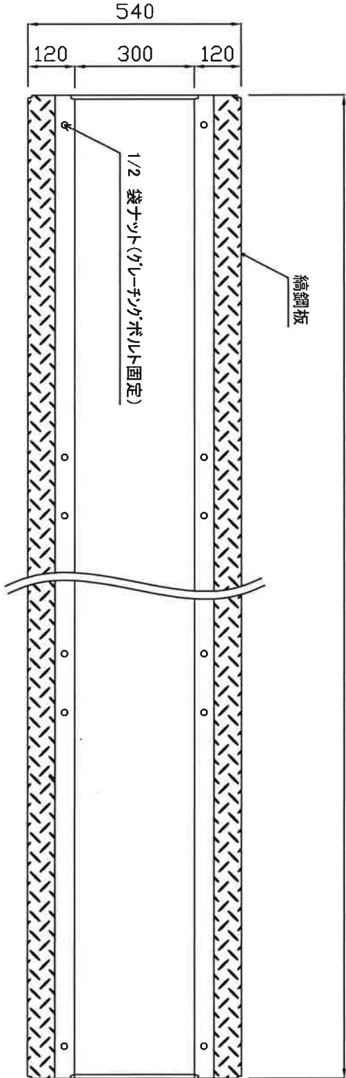
上面図
