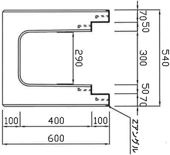
断面図
