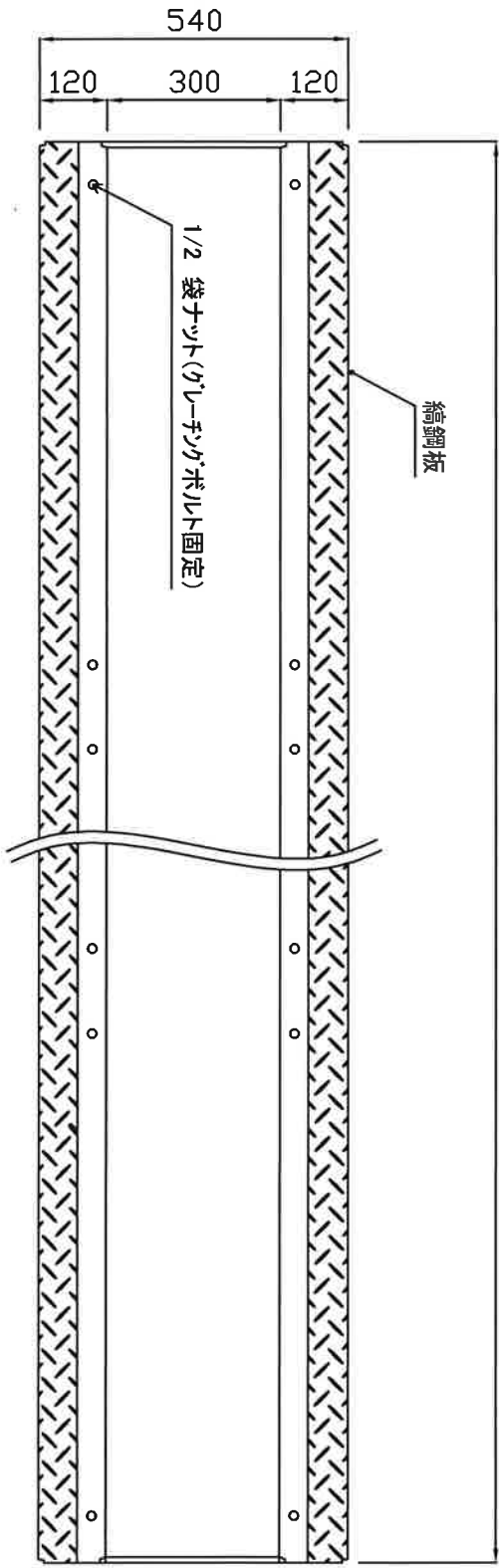
上面図
