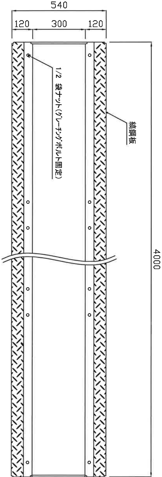
上面図
